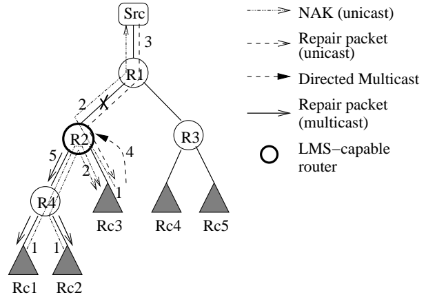
Fig. 3. LMS example
